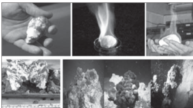
Рис. 3.21. Внешний вид газогидратов
