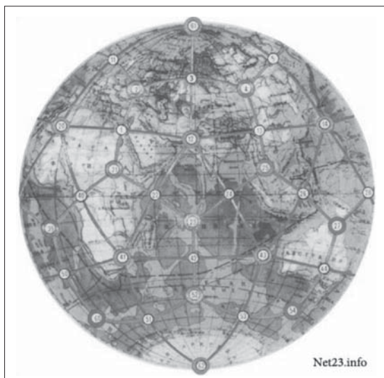
Рис. 2.16. Поверхностная решетка земного кристалла
