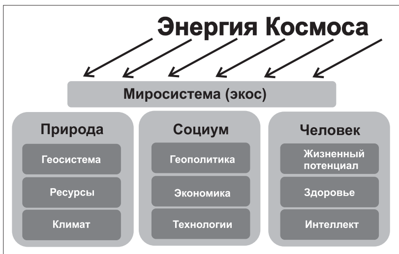
Рис. 1.1. Энергетическое воздействие космоса на социоприродную среду
