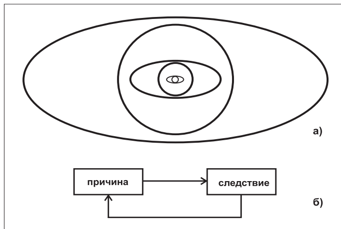
Рис. 1.2. Принцип бутстрапа: а - «все - во всем», б - причина - следствие
