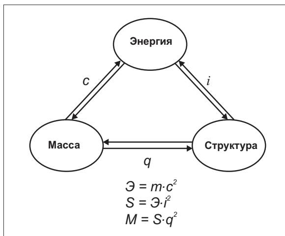
Рис. 1.4. Масса – энергия – структура
