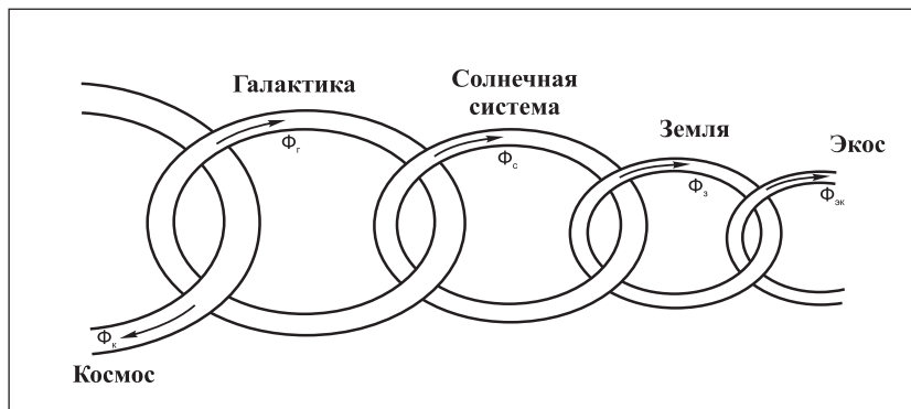
Рис. 1.8. Схема электромагнитного взаимодействия во Вселенной
