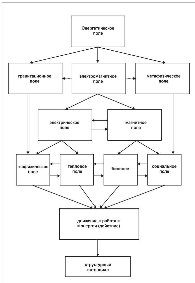
Рис. 1.6. Энергетическое поле, его разновидности и трансформации
